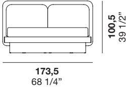
P24 con contenitore / P24 with storage unit
